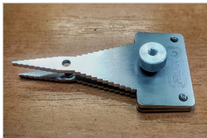
OH001 – Ohýbačka drátků
